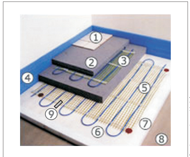
1 - Technischer Aufbau einer Elektro-Fußbodenspeicherheizung
